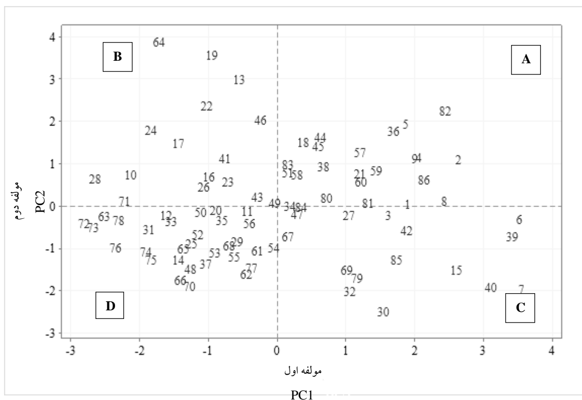
شکل ۲- نمودار بای پلات صفات و ژنوتیپ‌های بادمجان بر اساس دو مؤلفه‌های اول و دوم. (شماره‌های ۱ تا ۸۶ نشان دهنده ژنوتیپ‌های بادمجان مورد مطالعه در جدول ۱ است)
